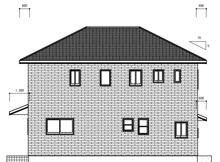
北立面図 1/100
