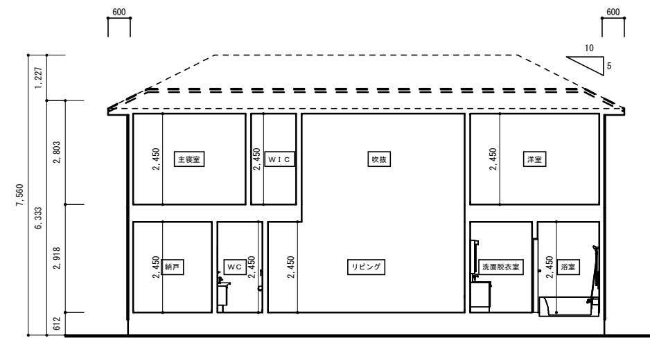
Y-Y' 断面図 1/100
