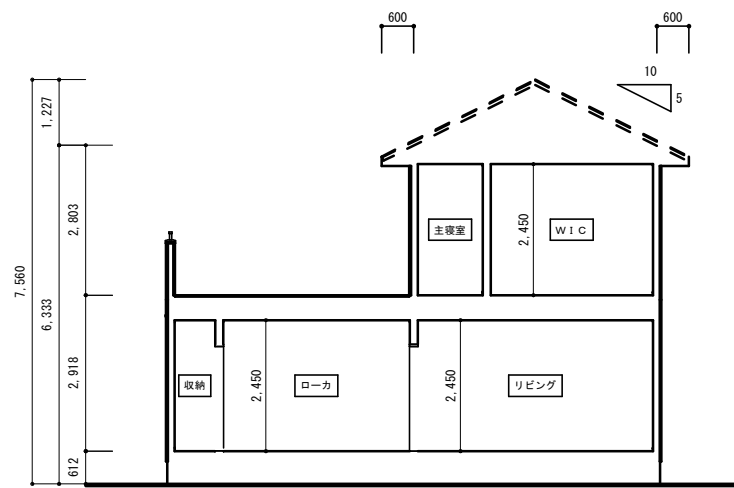
X-X' 断面図 1/100
